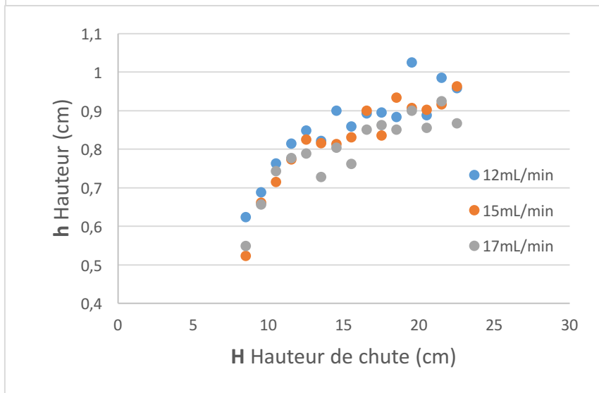
FIGURE 2 - (a) i. Courbe d'évolution de la section du fil à l'arrivée sur l'enroulement en fonction de la hauteur H d'écoulement pour un débit fixé (15 mL/min) ii. Courbe de compression d'une bulle dans le filet en fonction de sa distance au point de compression (b) Evolution de la hauteur moyenne de l'enroulement h en fonction de la hauteur de chute H pour différents débits sur plat (c) Evolution de la largeur moyenne de l'enroulement L en fonction de la hauteur de chute H pour différents débits sur plat
