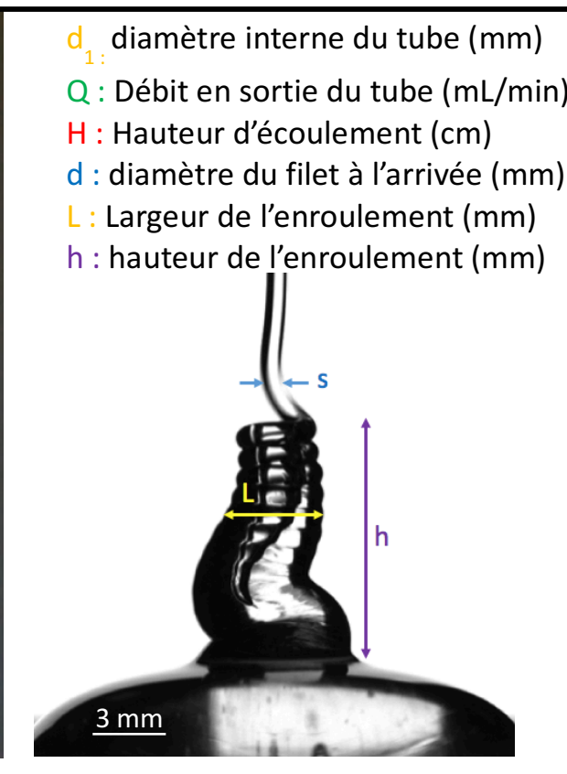
FIGURE 1 - (a) Schéma du dispositif expérimental (b) Paramètres mesurés sur l'instabilité (c) Différents régimes d'instabilité observés 1. Régime sans instabilité 2. Régime d'enroulement simple 3. Régime de surenroulement 4. Régime à haute instabilité
