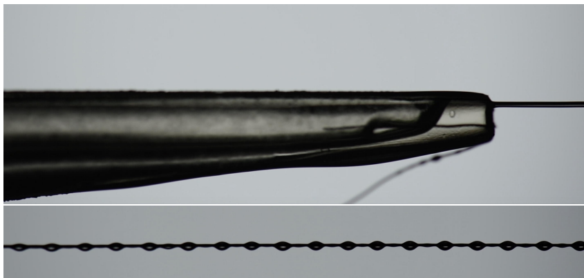
FIGURE 1 – Dépôt d'un film de liquide visqueux sur un fil métallique (en haut). Gouttes apparaissant sur le fil après quelques s. (en bas)
