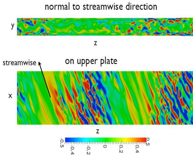
Figure2. a) Moyenne temporelle de la vorticité longitudinale sur la plaque supérieure, la plaque inférieure, et dans un plan entre les deux plaques. b) vorticité longitudinale instantanée sur la plaque supérieure et sur un plan entre les deux plaques. Les tourbillons longitudinaux (“streamwise vortices”) et stries (“streaks”) sont évidents près des plaques.
