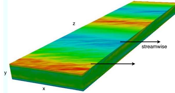
Figure1. Visualisation 3D de la vorticité longitudinale de l'écoulement moyen. Le domaine entier, de dimensions L_x \times L_y \times L_z = 10 \times 2 \times 40 est montré. Les bandes sont parallèles à la direction x , tandis que les petites structures ("streaks") sont alignées dans la direction longitudinale ("streamwise") qui est orienté à un angle de 24^\circ à la direction x .
